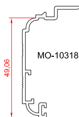
پروفیل روکوب شیاردار
