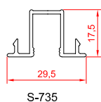
زهوار تک جداره
