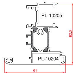
پروفیل وسط دو لنگه
