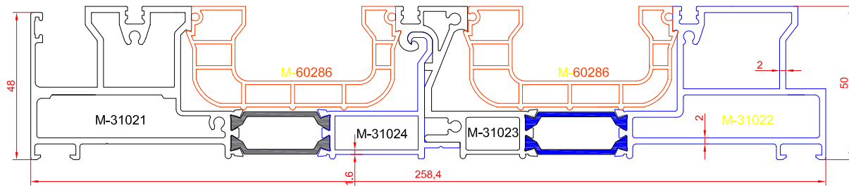
آداپتور فریم سه ریل
