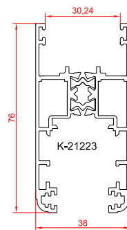
پروفیل لنگه بدون زهوار جدید
