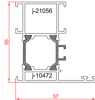
پروفیل فریم
