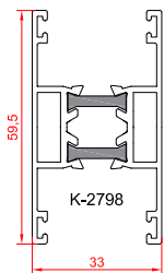
پروفیل سپری بدون زهوار
