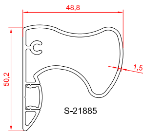
دستگیره کششی
