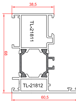
پروفیل فریم
