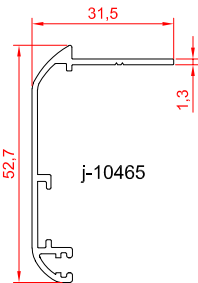
پروفیل روکوب ۵۲
