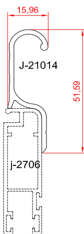
دستگیره لنگه توری
