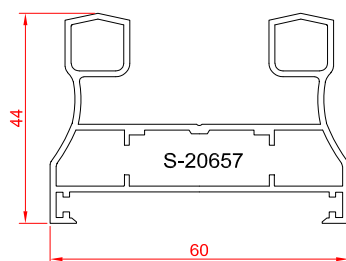
پروفیل فریم جدید
