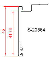
پروفیل روکوب
