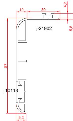
روکوب ۸۷ میلی متری
