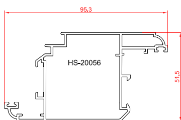
پروفیل لنگه
