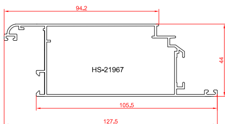
لنگه بلند درب
