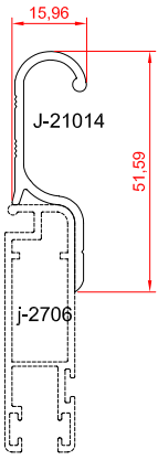
دستگیره لنگه توری
