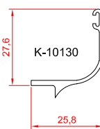
ریل توری
