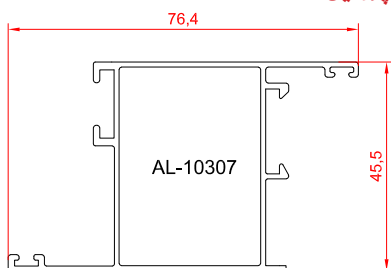
پروفیل لنگه
