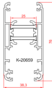
پروفیل بدون زهوار
