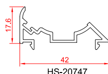
پروفیل گردان فریم
