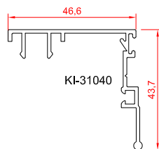
درپوش سپری بازشو لولایی
