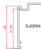
پروفیل روکوب
