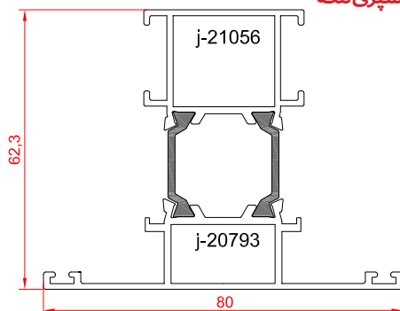
پروفیل سپری لنگه
