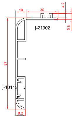
روکوب ۸۷ میلی متری
