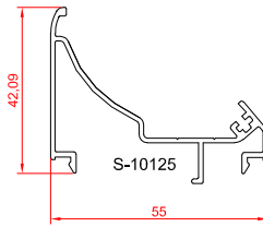
پروفیل گردان فریم
