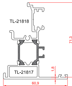
پروفیل مابین دو لنگه
