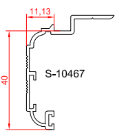
روکوب ۴۲
