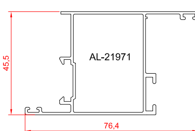
لنگه الدوکس با ضخامت ۲ میلی متر
