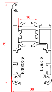
پروفیل لنگه زهوار دار
