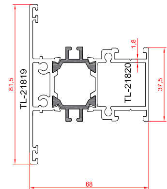
پروفیل سپری
