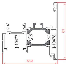
پروفیل وسط دو لنگه
