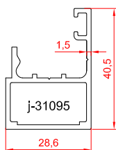
پروفیل جان پناه
