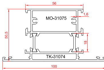
سپری کتیبه پایین
