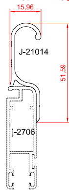
دستگیره لنگه توری
