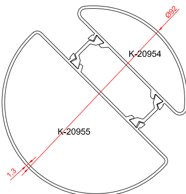
لوله محوری ترمال بریک
