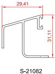
کاور فریم
