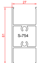
پروفیل سپری
