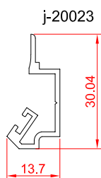
پروفیل گردان فریم
