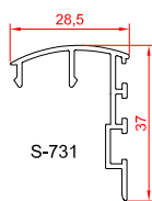
درپوش لنگه ی ۷۳۱
