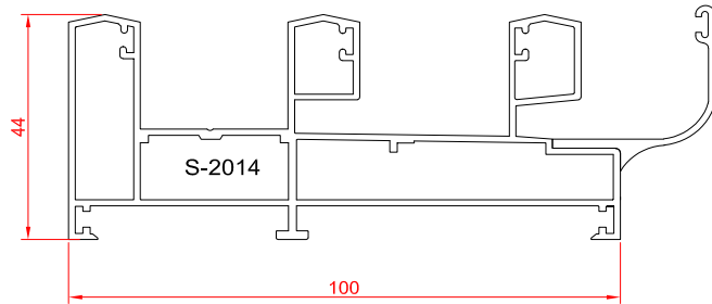
پروفیل فریم سه ریل
