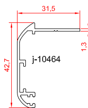
پروفیل روکوب ۴۲
