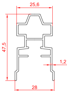
پروفیل لنگه بازشو
