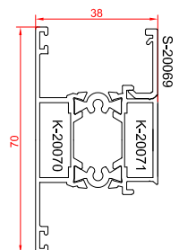
پروفیل سپری ۲۱۲۲۳
