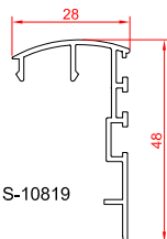
درپوش لنگه های ۲۱۳۴۰
