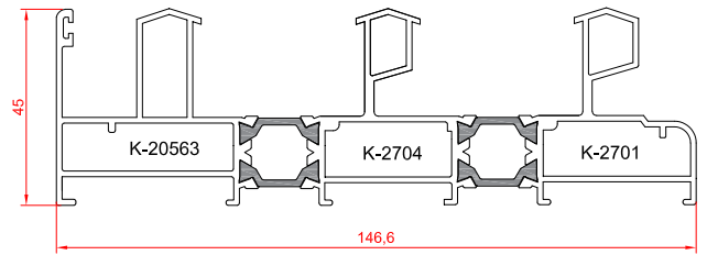
پروفیل فریم سه ریل
