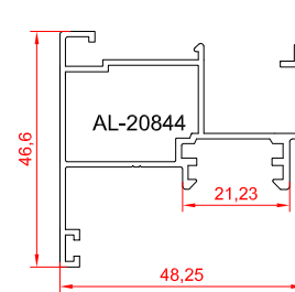
پروفیل وسط دو لنگه
