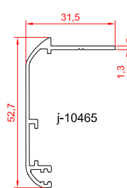
پروفیل روکوب ۵۲
