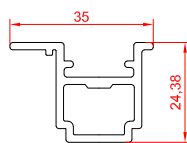
پروفیل آداپتوری و جای تسمه
