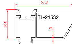
پروفیل آداپتور زهوار فیکس بازشو مخفی
