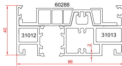
آداپتور چهارلنگه وسط بازشو
