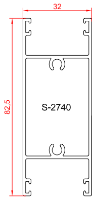
پروفیل سپری بدون زهوار
