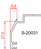
پروفیل روکوب ۳ سانتی
