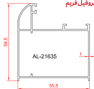
پروفیل فریم
