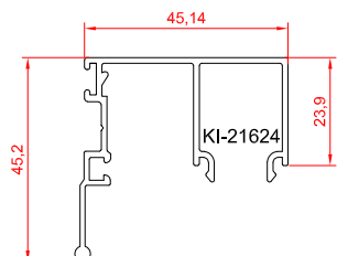
اینترلاک در سپری فریم
