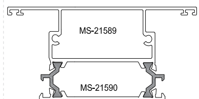
پروفیل سپری لنگه
