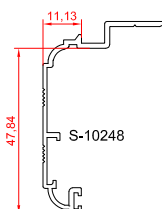
پروفیل روکوب شیاردار
