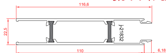
ورق دو جداره ترمال بریک
