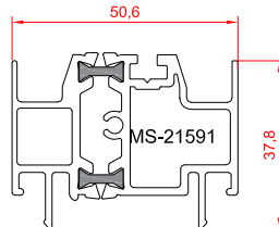
پروفیل وسط چهارلنگه
