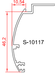
پروفیل روکوب گرد شیاردار
