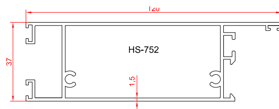
پروفیل پایین درب
