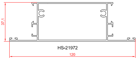
سپری بلند لولایی
