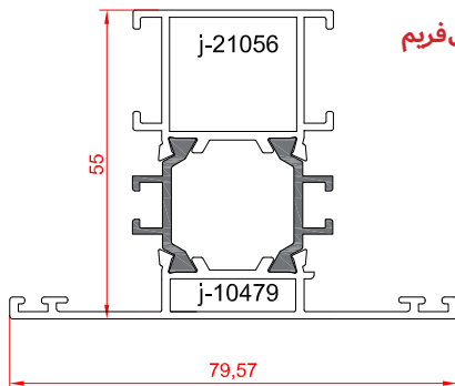
پروفیل سپری لنگه
