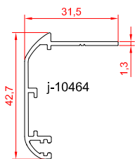
پروفیل روکوب ۴۲
