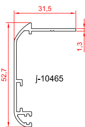
پروفیل روکوب ۵۲
