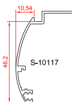
پروفیل روکوب گرد شیاردار
