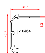
پروفیل روکوب ۴۲
