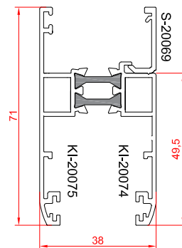
پروفیل لنگه بازشو کشویی
