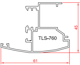
پروفیل وسط دولنگه
