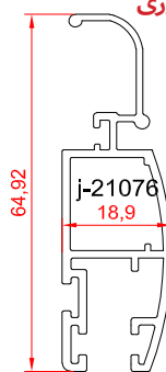
لنگه توری
