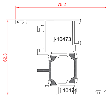
لنگه پنجره
