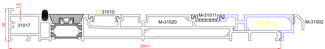
فریم دفنی سه ریل
