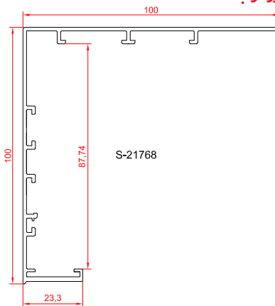
روکوب ۱۰*۱۰
