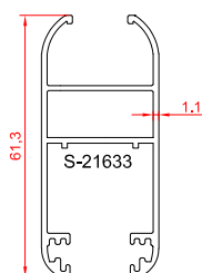
لنگه تک جداره
