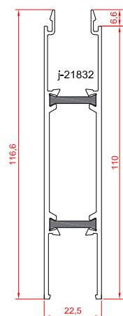
ورق دو جداره ترمال بریک
