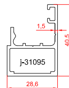
پروفیل جان پناه
