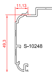
پروفیل روکوب شیاردار
