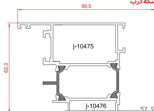
لنگه درب
