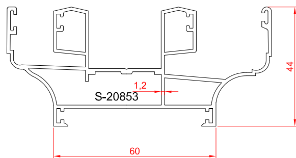
پروفیل فریم دارای عرق گیر
