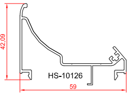
پروفیل گردان فریم
