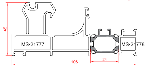
پروفیل فریم مونوریل
