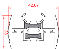
پروفیل وسط چهار لنگه
