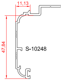
پروفیل روکوب شیاردار
