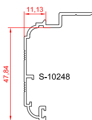
پروفیل روکوب شیاردار
