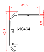
پروفیل روکوب ۴۲
