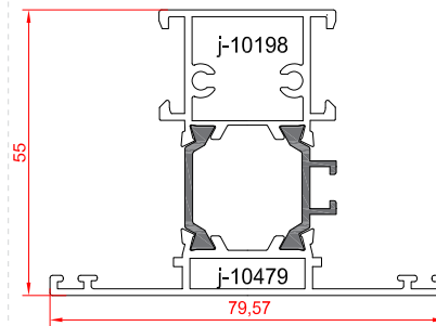
پروفیل سپری فریم
