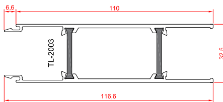
ورق دوجداره ترمال بریک
