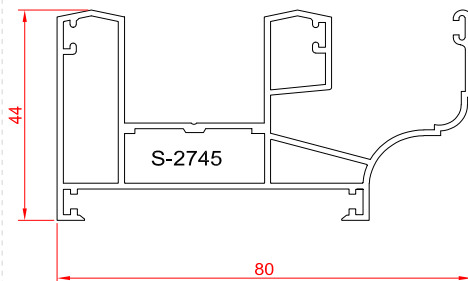
پروفیل فریم ریل دار
