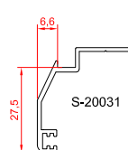
پروفیل روکوب ۳ سانتی
