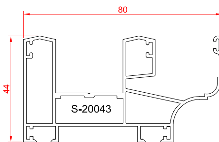
پروفیل فریم پایین لاستیک خور
