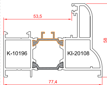
پروفیل کتیبه
