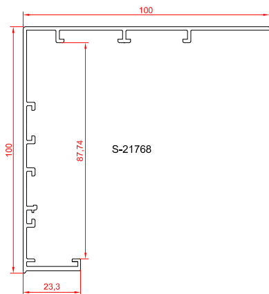
روکوب ۱۰*۱۰ میلی متری
