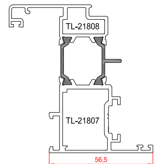
پروفیل لنگه پنجره
