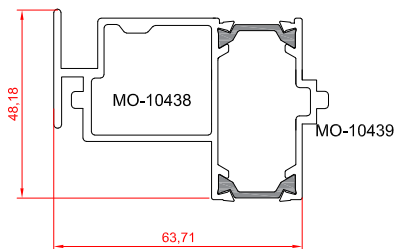
پروفیل وسط چهار لنگه
