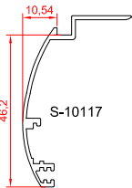
پروفیل روکوب گرد شیاردار
