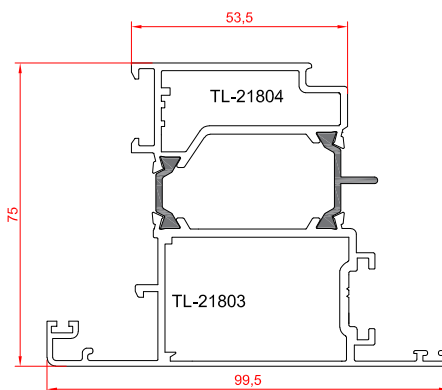
لنگه درب بیرون بازشو
