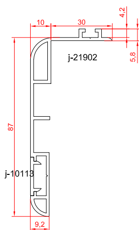
روکوب ۸۷ میلی متری
