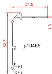
پروفیل روکوب ۵۲
