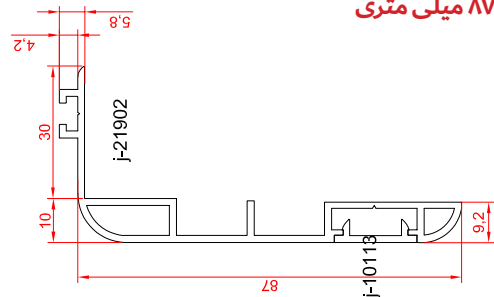
روکوب ۸۷ میلی متری
