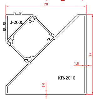
آداپتور کنج فریم
