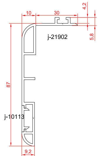
روکوب ۸۷ میلی متری
