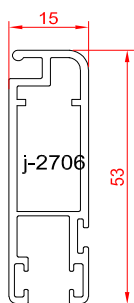
لنگه توری
