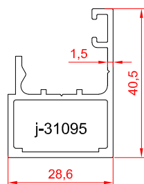
پروفیل جان پناه
