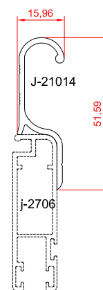
دستگیره لنگه توری
