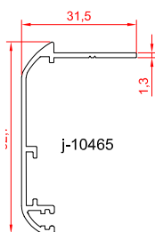
پروفیل روکوب ۵۲
