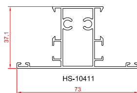
پروفیل سپری
