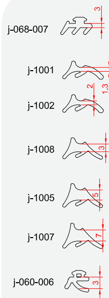
thermal break hinged door
