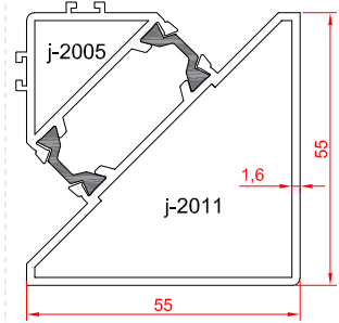
آداپتورکنج فریم
