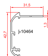
پروفیل روکوب ۴۲
