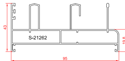
پروفیل فریم
