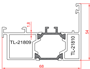
آداپتور درب بیرون بازشو
