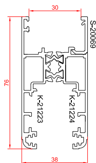
پروفیل لنگه زهوار دار
