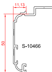
روکوب ۵۲
