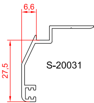
پروفیل روکوب ۳ سانتی
