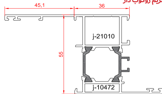
فریم روکوب دار
