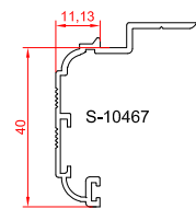
پروفیل روکوب
