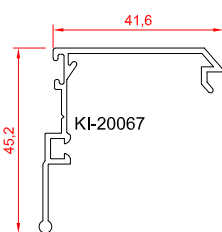
اینترلاک لنگه
