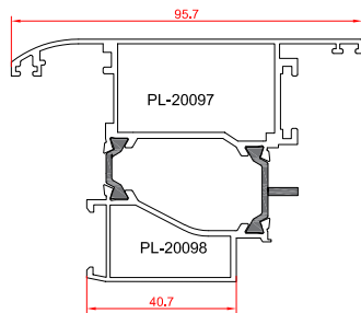
پروفیل لنگه بیرون بازشو درب
