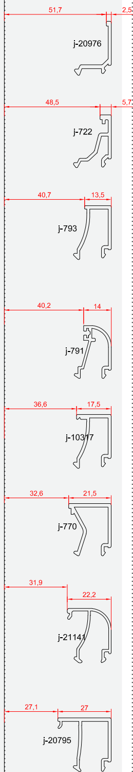
thermal break hinged door
