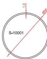
لوله محوری ۶۰
