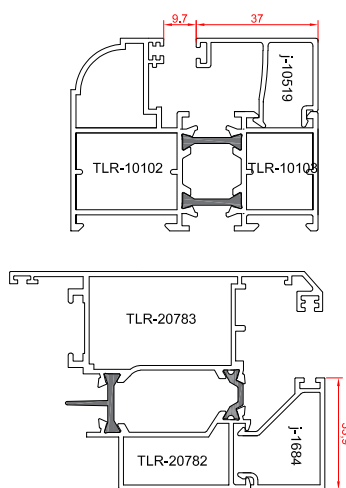
thermal break hinged door
