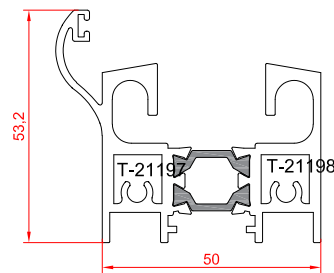
bottom frame guide 1.996 kg/m
