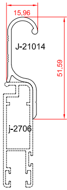
دستگیره لنگه توری
