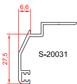
پروفیل روکوب ۳ سانتی
