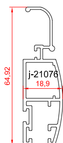
لنگه توری
