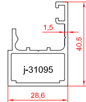
پروفیل جان پناه
