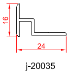
پروفیل مابین دو فریم
