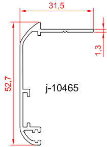
پروفیل روکوب ۵۲
