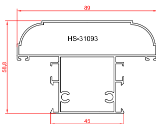
پروفیل سپری جدید
