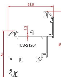
پروفیل لنگه
