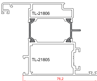
لنگه درب داخل بازشو
