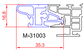
پروفیل اینترلاک
