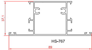
پروفیل سپری
