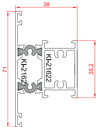
سپری برای فریم مونوریل
