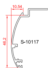
پروفیل روکوب گرد شیاردار
