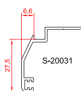
پروفیل روکوب ۳ سانتی
