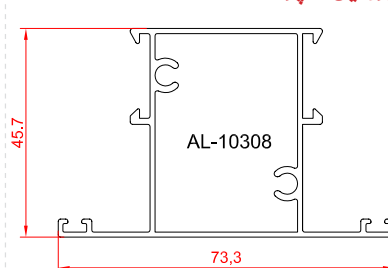
پروفیل سپری
