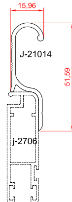
دستگیره لنگه توری
