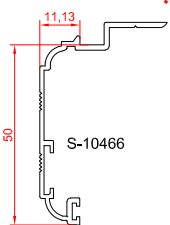
روکوب ۵۲
