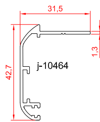
پروفیل روکوب ۴۲
