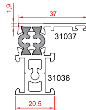
سپری بازشو لولایی
