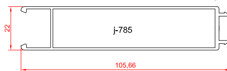
ورق دو جداره
