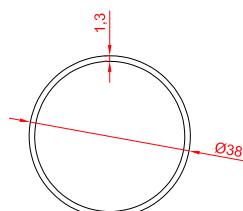
لوله محوری ۳۸
