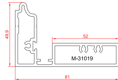
آداپتور سه لنگه وسط بازشو
