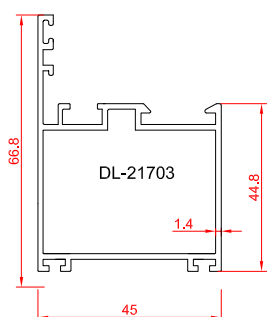
فریم و لنگه بازشو بادبزی
