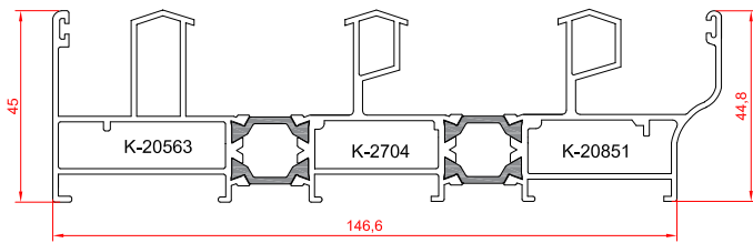
پروفیل فریم سه ریل
