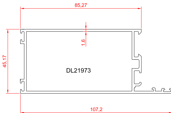
فریم تخت و بلند بادبزی
