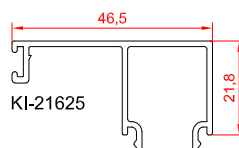
درپوش مونوریل
