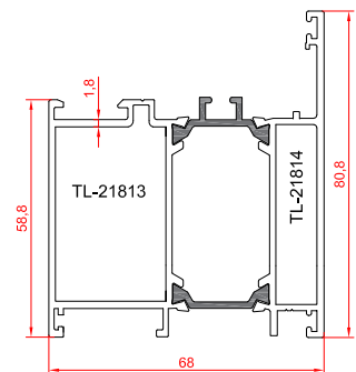
فریم درب
