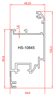
لنگه یراق یوپوی سی ضخامت ۱۰۶
